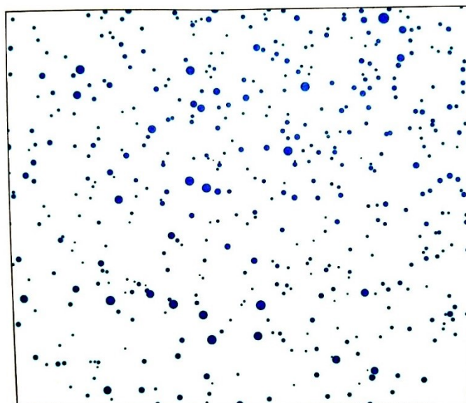
Рис. 17. Немая карта участка неба
